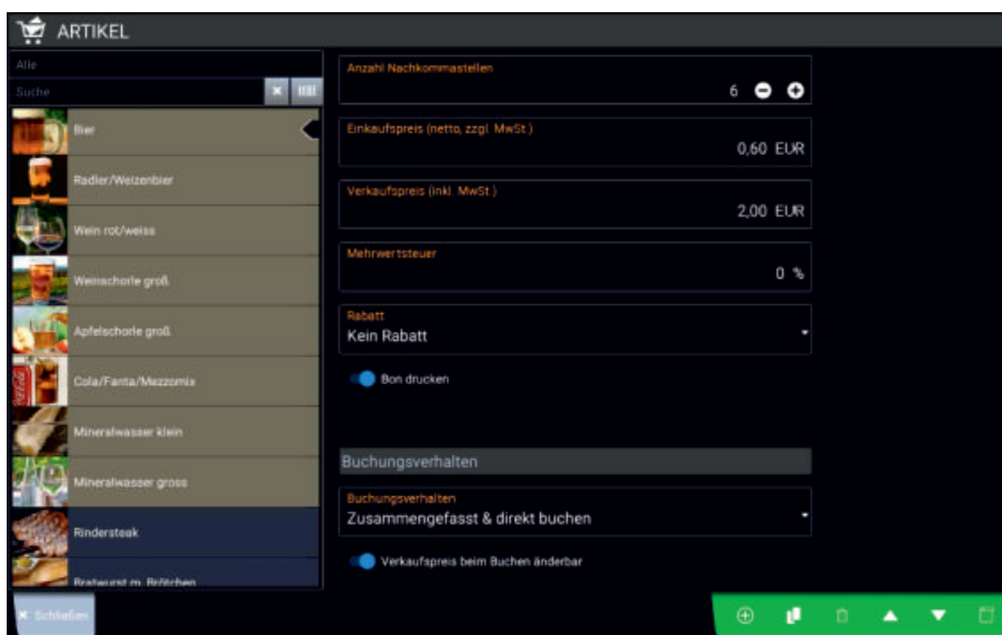
Artikelverwaltung
